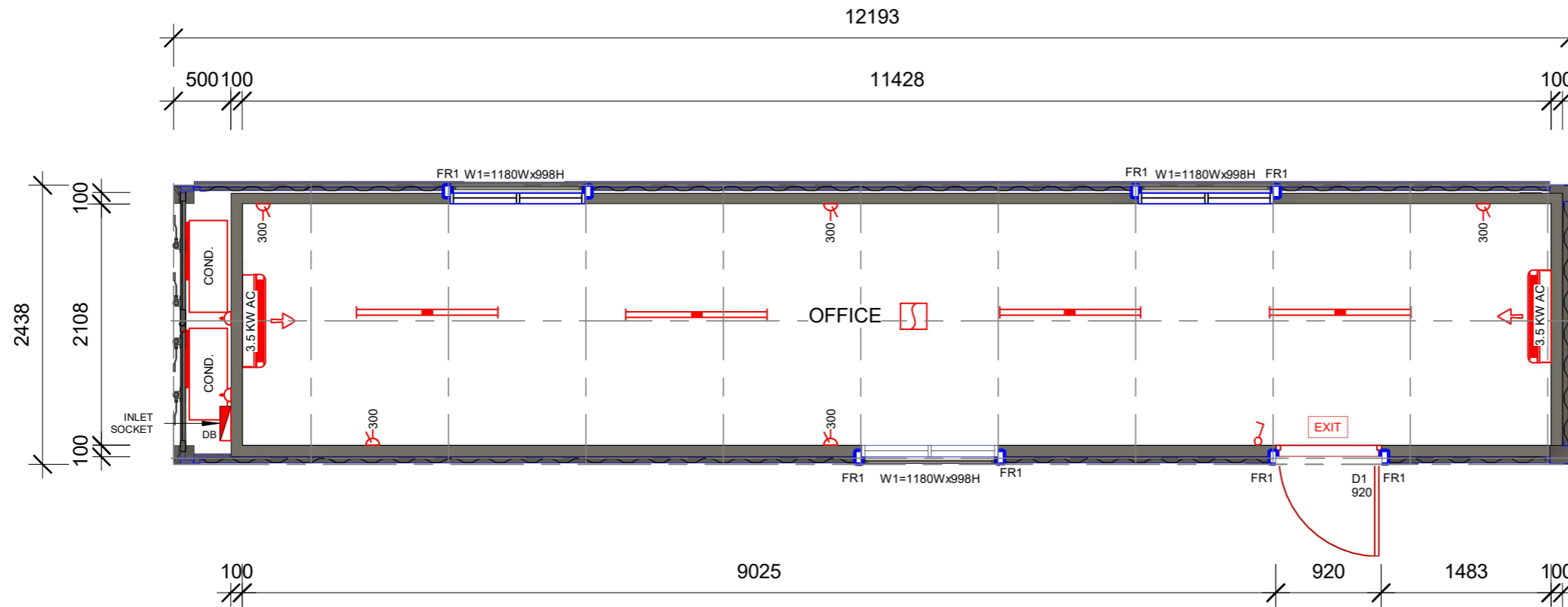
1 FLOOR PLAN 1 : 50
