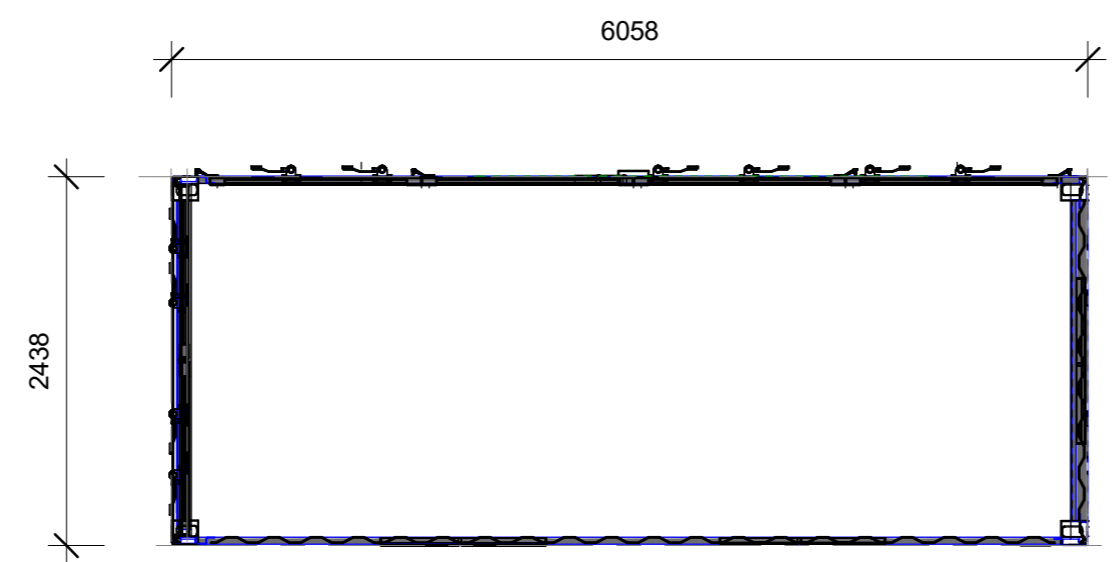
1 FLOOR PLAN 1 : 50
