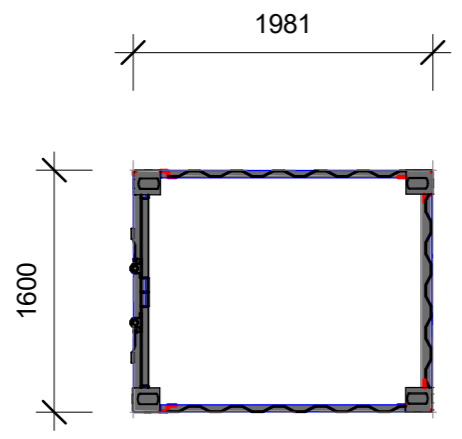
1 FLOOR PLAN 1 : 50
